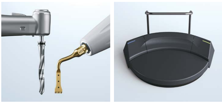
Länk mellan Surgic Pro2 och VarioSurg 4
